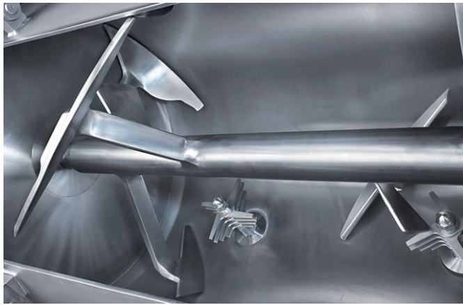
Pflugschar®-Chargenmischer mit modifiziertem Schleuderwerk
