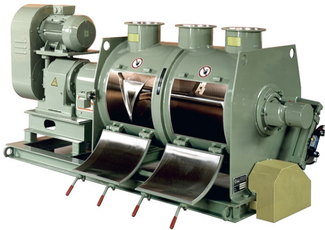
Pflugschar®-Chargenmischer FKM 600 D
